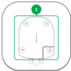
2 - Plaque de montage de SmartBracket (glissez de force vers le bas pour ouvrir ; une section perforée est nécessaire pour déclencher l'inviolabilité lors des tentatives d'arrachement du hub de la surface)
