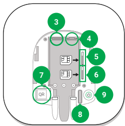
3 - Connecteur de câble d'alimentation 4 - Connecteur Ethernet 5 - Connecteur 2: carte SIM de sauvegarde (format micro-SIM) 6 - Connecteur 1: carte SIM principale (format micro-SIM) 7 - Code QR 8 - Bouton anti-sabotage 9 - Bouton de mise en marche
