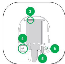
3 - Connecteur d'alimentation 4 - Code QR 5 - Bouton anti-sabotage 6 - Bouton de mise en marche
