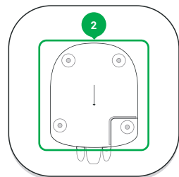
2 - Plaque de montage SmartBracket (une section perforée est nécessaire pour déclencher l'autoprotection lors d'une tentative de soulèvement de ReX de la surface)
