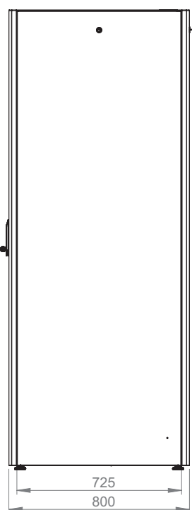
Vue latérale
