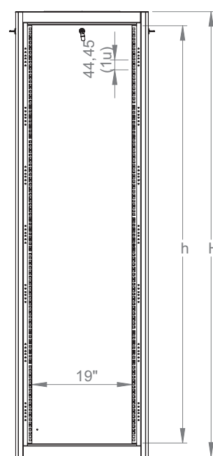
Dimensions en largeur et hauteur
