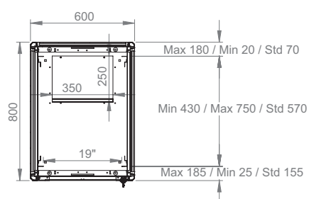
Équipement Max/Std/Min distance de montage
